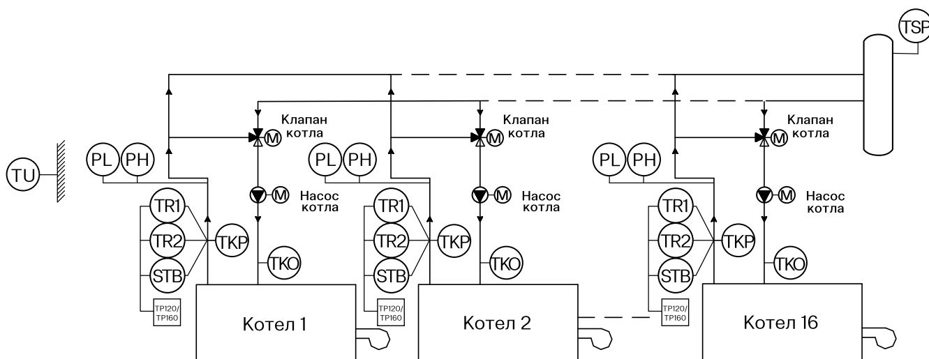
Рис. 20. Функциональная схема котлоагрегата и его компонентов
