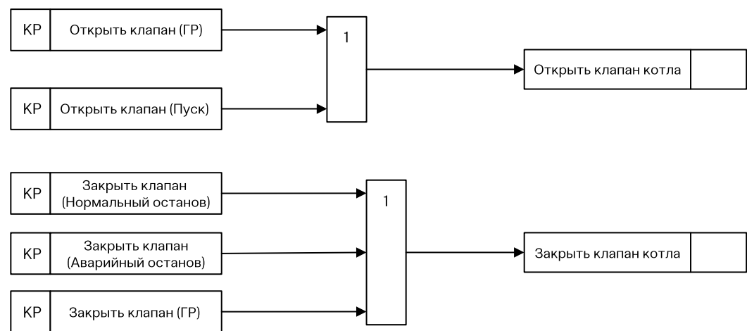
Рис. 19. Алгоритм управления клапаном котла
