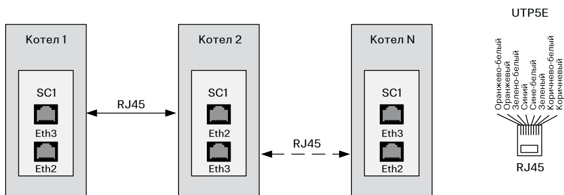
Подключение котлов в систему каскадного управления
