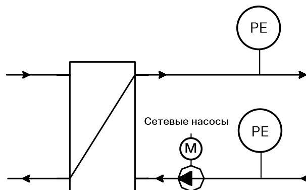
Рис. 24. Конфигурация 4. Автоматическое управление КА и частотное управление сетевыми насосами (поддержание заданного перепада давления между прямой и обраткой)
