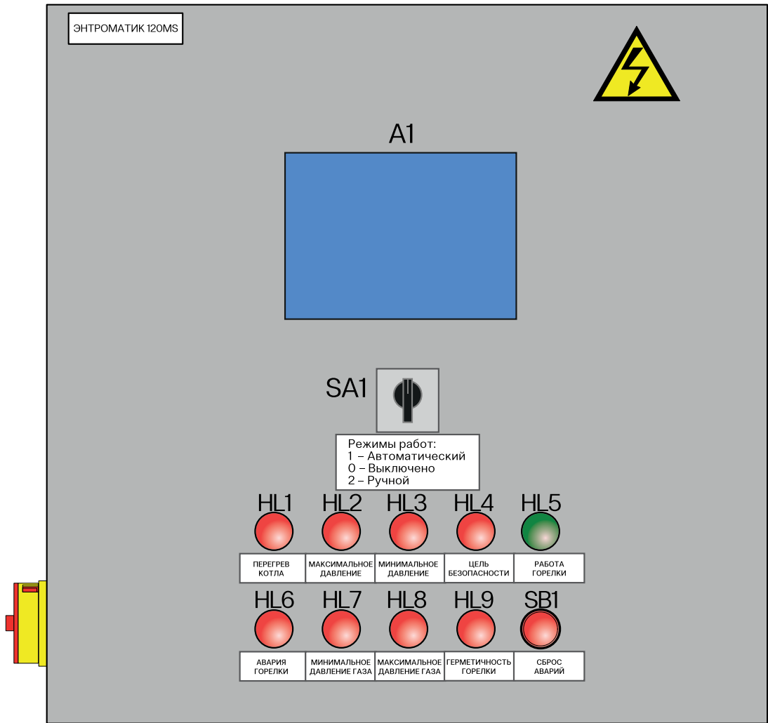
Рис. 1. Внешний вид щита
