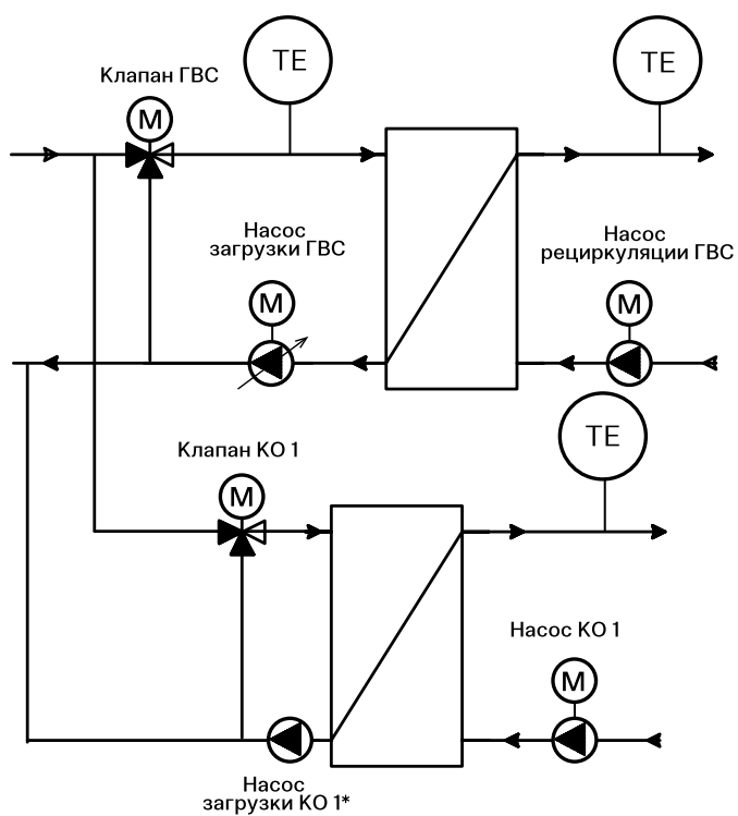
Рис. 25. Конфигурация 5. Автоматическое управление КА и одним контуром отопления и контуром ГВС
