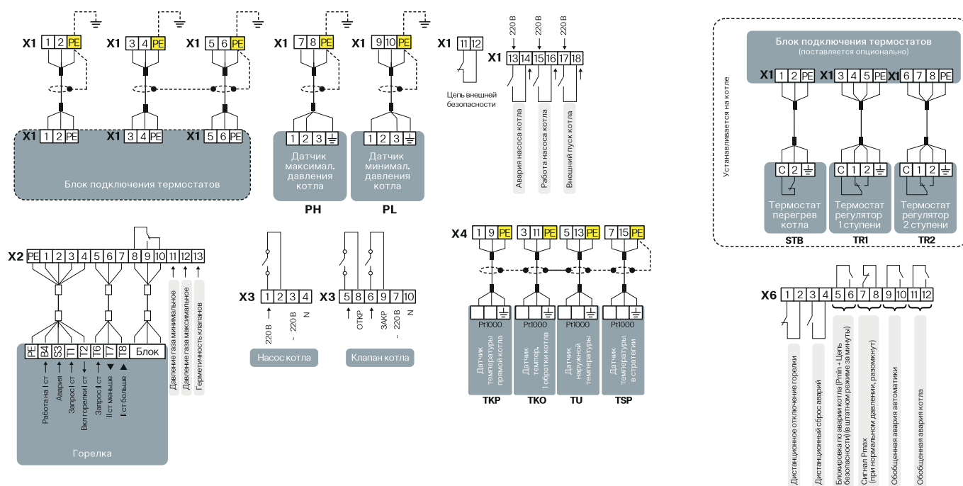
Конфигурация 1: 2 КО, нет ГВС, нет подпитки, нет сетевых насосов
