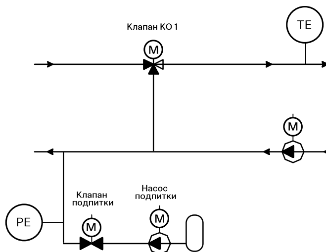
Рис. 22. Конфигурация 2. Автоматическое управление КА и одним контуром отопления и возможностью автоматической подпитки
