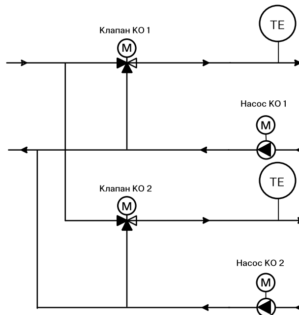
Рис. 21. Конфигурация 1. Автоматическое управление КА и двумя контурами отопления
