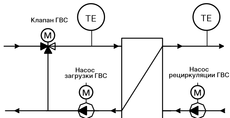
Рис. 23. Конфигурация 3. Автоматическое управление КА и контуром ГВС
