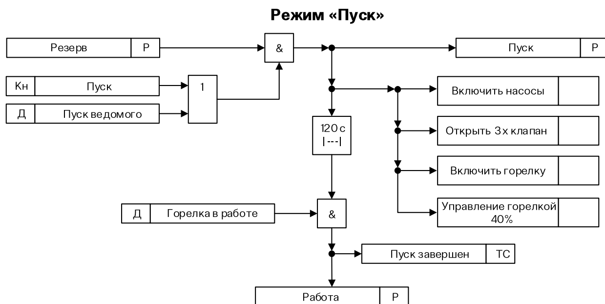
Рис. 14. Алгоритм режима «Пуск»
