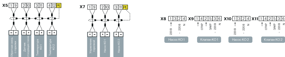
Конфигурация 2: 1 КО, нет ГВС, есть подпитка, нет сетевых насосов
