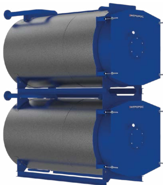
Общий вид двухкотловой установки
