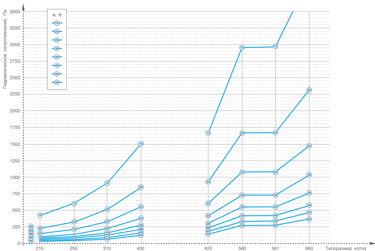
Зависимость гидравлического сопротивления котлов ТТ50 от Δt
