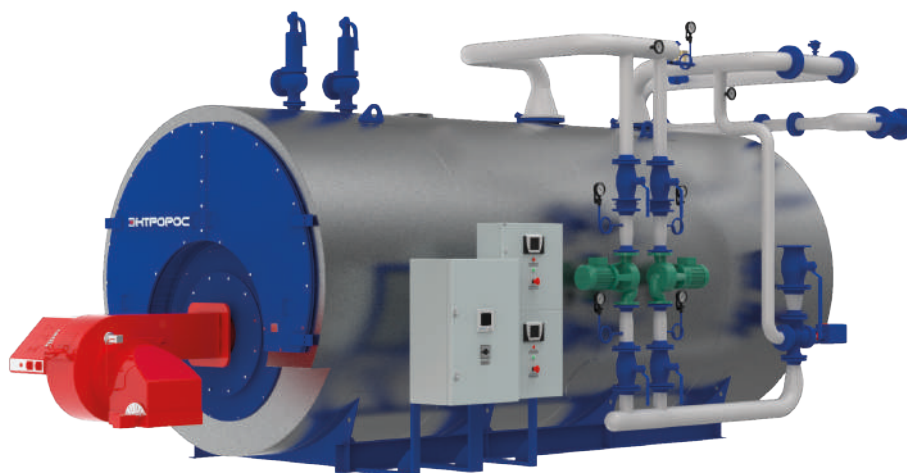
Котлоагрегат на базе котла ТТ150
