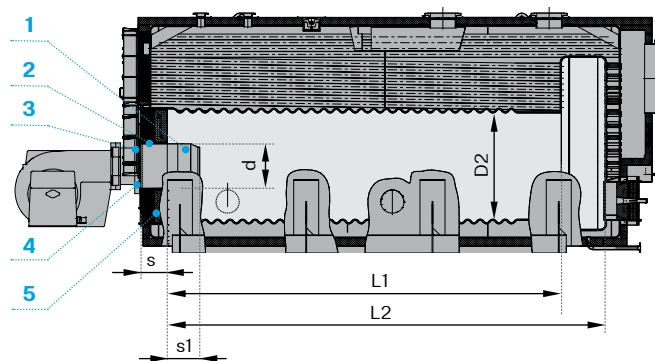
Установка горелки
