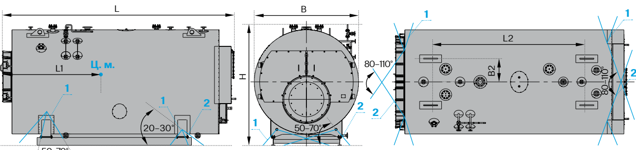
Схема транспортировки котла
