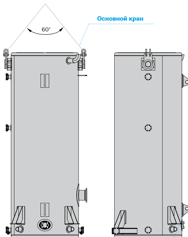
Строповка конвективной части
