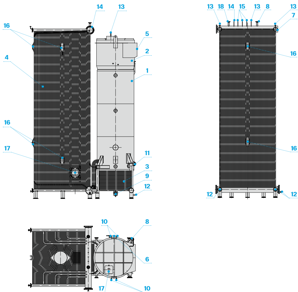
Конструктивная схема котла ТТ300
