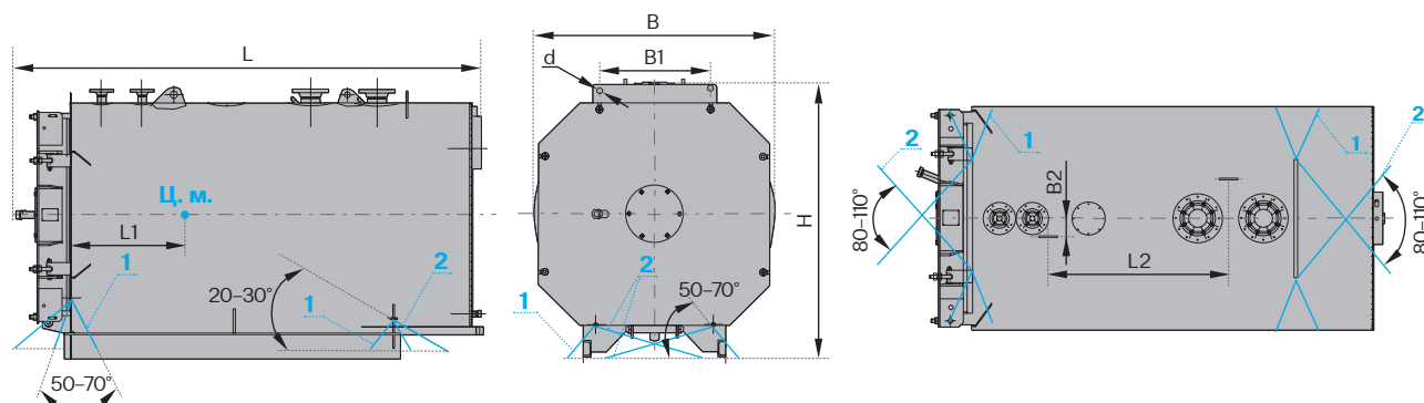
Схема транспортировки котла
