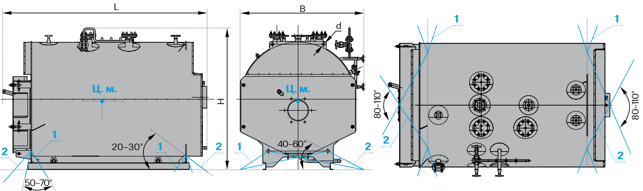
Схема транспортировки котла
