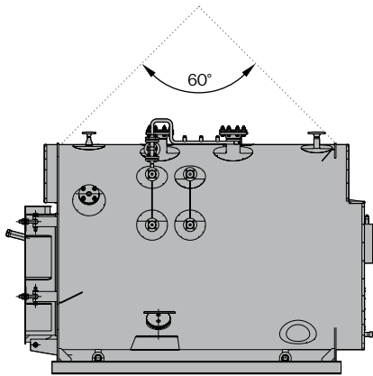
Принципиальная схема строповки котла
